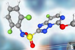
Florasulam
